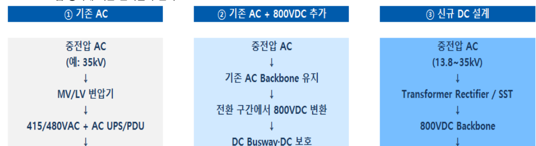
800VDC 도입 방식에 따른 전력설비 변화
